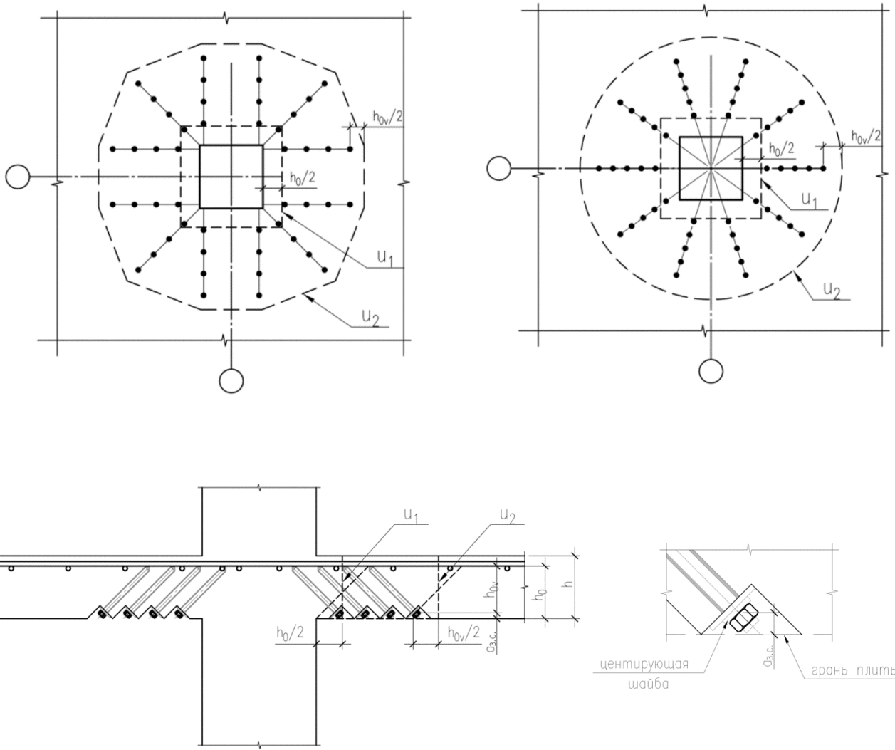
Рисунок 5.1. Периметры расчетных сечений.
