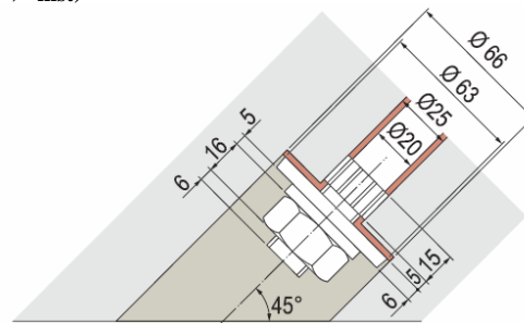
Головная часть анкера и расширение отверстия HZA-P M20
