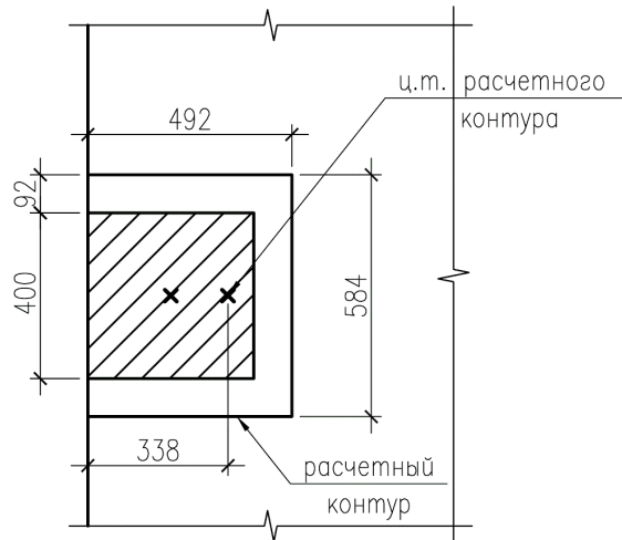
Рисунок А1. Расчетная схема на продавливание без поперечного армирования.
