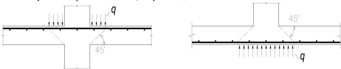
Рисунок 5.4. Разгружающие усилия при расчете на продавливание.
