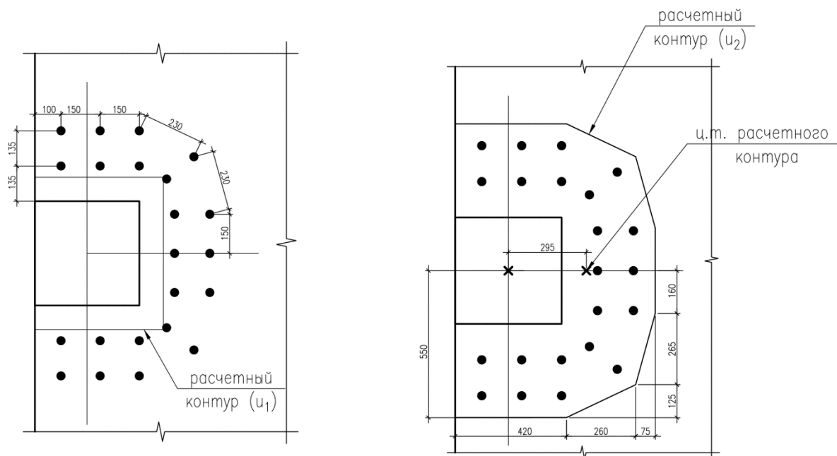
Рисунок А3. Расчетная схема за контуром поперечной арматуры Hilti HZA-P.
