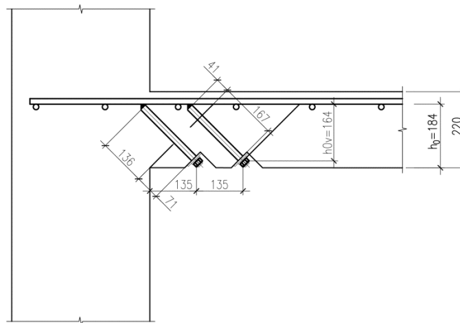
Рисунок А2. Схема установки поперечной арматуры Hilti HZA-P.
