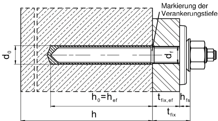
Bild A2: HAS-U... mit Hilti Verfüll-Set
