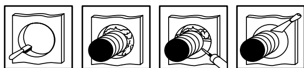
Герметизация трубных проходок
