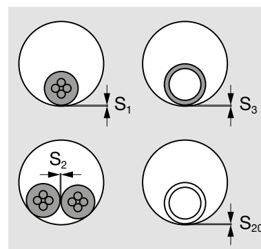
Рисунок А5. Расстояния внутри проема
