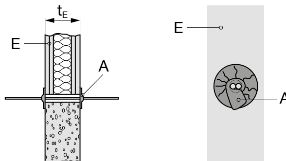
Рисунок А4. Установка противопожарного диска для прокладки кабелей Hilti CFS-D
