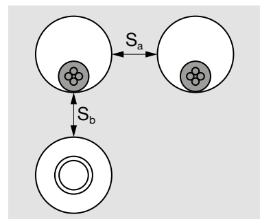
Рисунок А6. Расположение пучков кабелей
