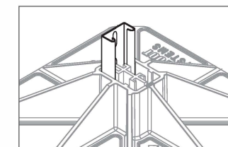
Взаимозаменяемая траверса 21 x41 x 15мм
