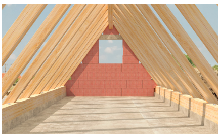
Крепления балок
