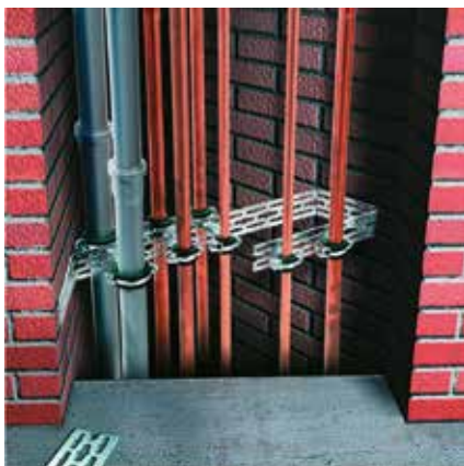
StaboFix® Фиксирующая пластина
