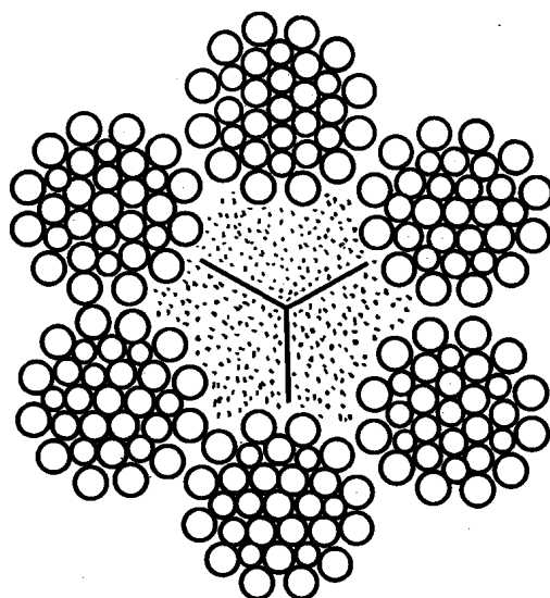
Шестипрядный канат 6 \times 31 + 1 о. с.; 6 \times 31 = 186 проволок с органическим сердечником (прясть каната 1 + 6 + 6/6 + 12 ).
